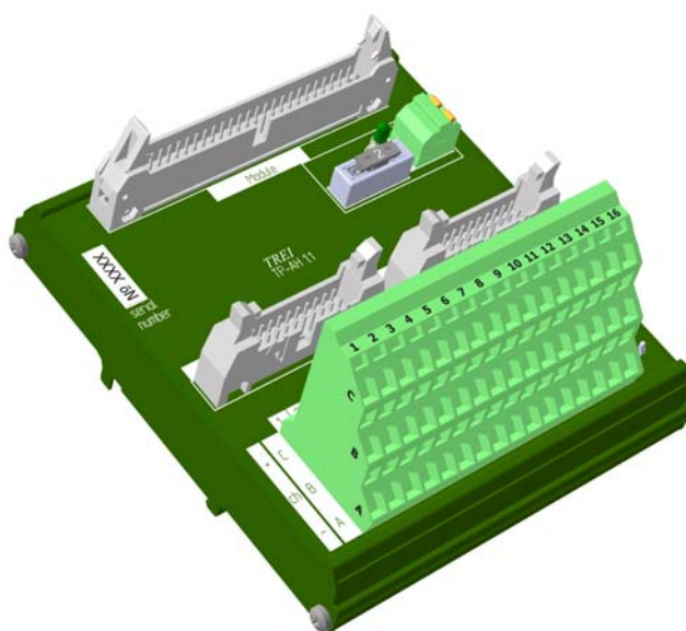
Рисунок 2 - Внешний вид терминальной панели аналогового ввода TP-AH
