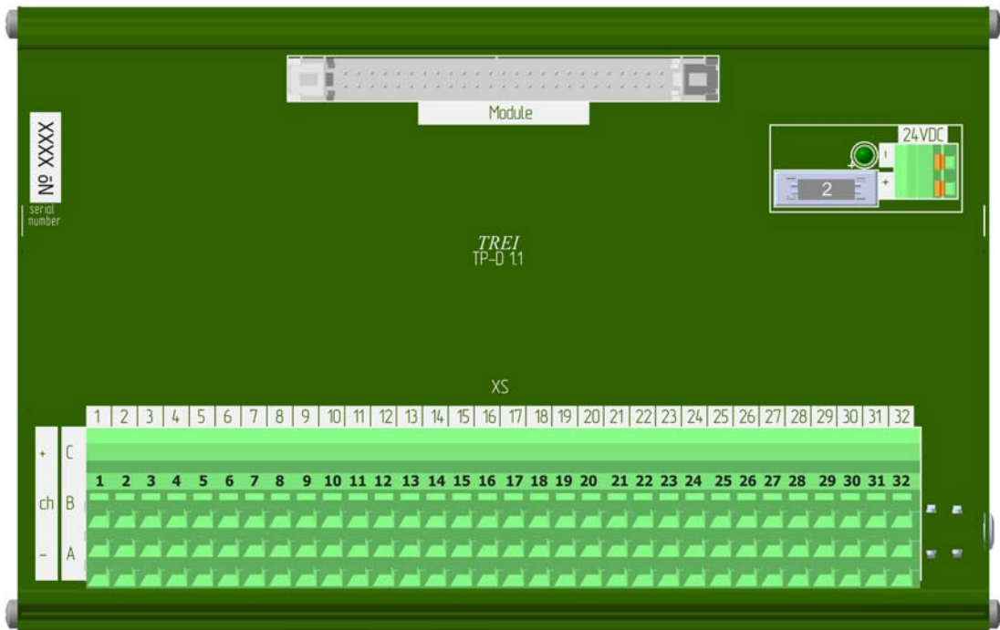
Рисунок 3 - Разъемы и лицевая панель терминальной панели TP-D
