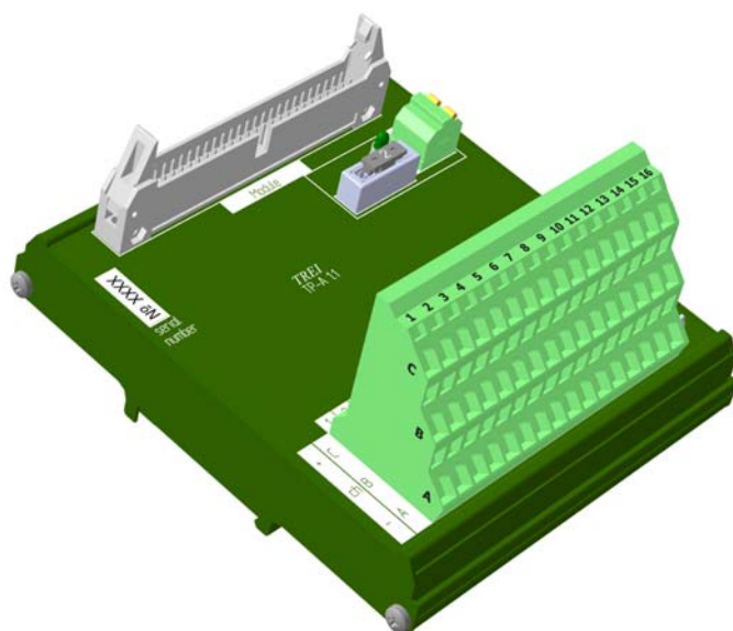
Рисунок 1 - Внешний вид терминальной панели аналогового ввода TP-A
