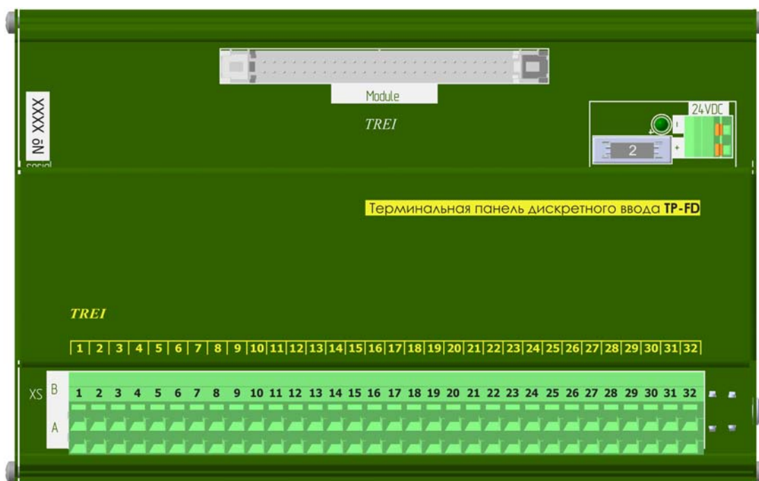
Рисунок 6 - Разъемы и лицевая панель терминальной панели TP-FD
