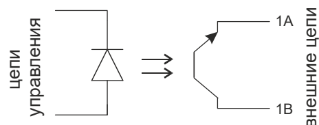
Рисунок 7 - Назначение контактов реле 1-го канала в TP-R2, TP-2R2
