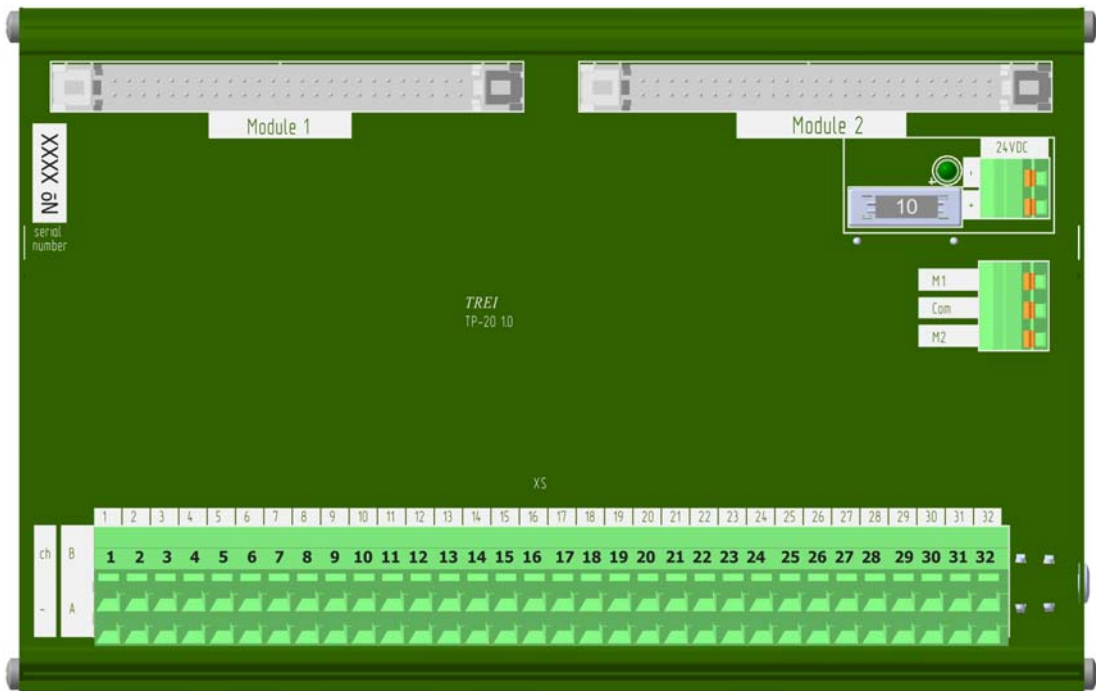
Рисунок 4 - Разъемы и лицевая панель терминальной панели TP-20
