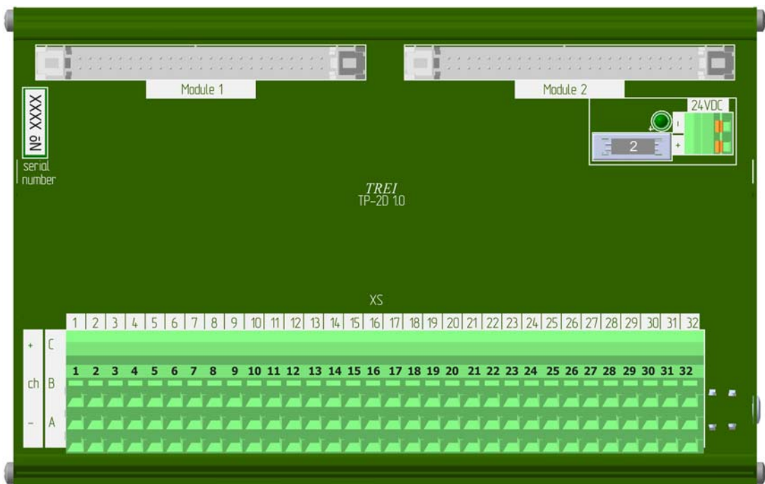
Рисунок 4 - Разъемы и лицевая панель терминальной панели TP-2D
