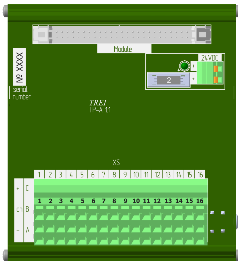
Рисунок 3 - Разъемы и лицевая панель терминальной панели TP-A
