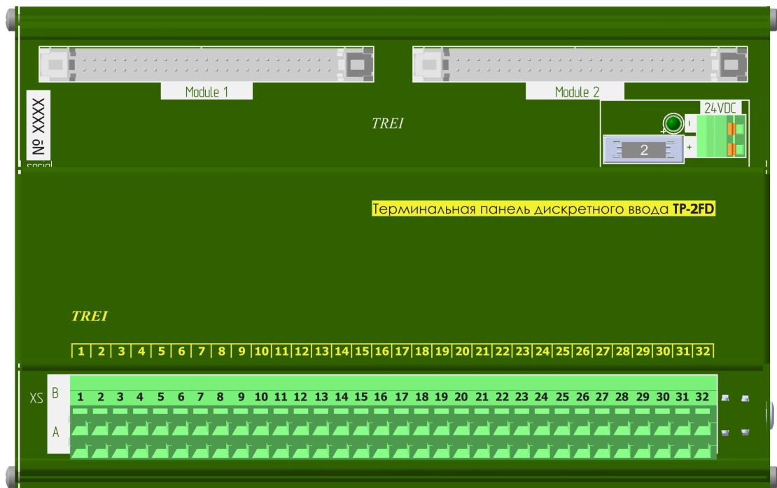
Рисунок 8 - Разъемы и лицевая панель терминальной панели TP-2FD
