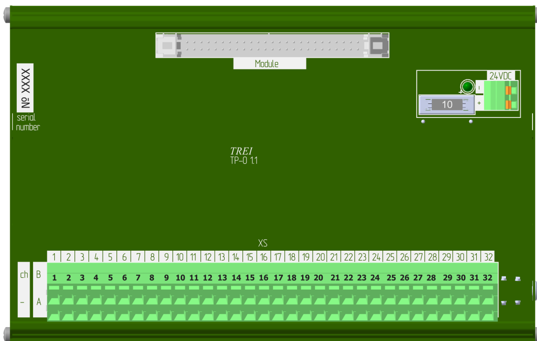
Рисунок 3 - Разъемы и лицевая панель терминальной панели TP-O
