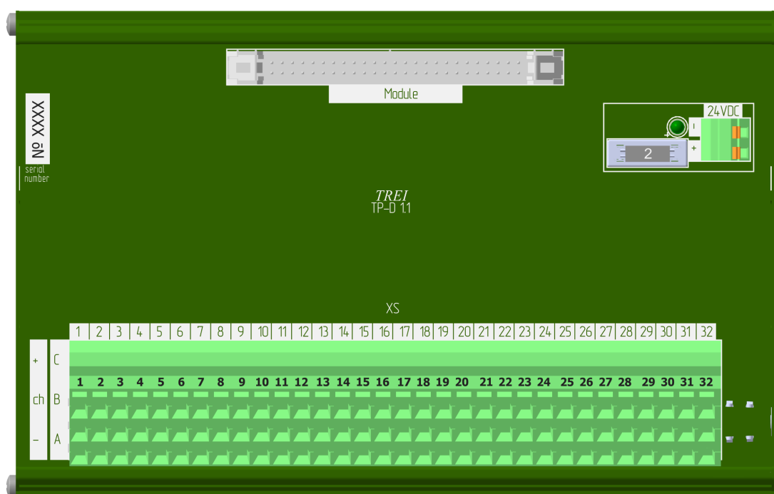
Рисунок 3 - Разъемы и лицевая панель терминальной панели TP-D
