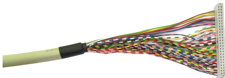
Рисунок 1 - Внешний вид кабеля CIDC с разъемом IDC-50, вариант выхода конца кабеля - прямой.
