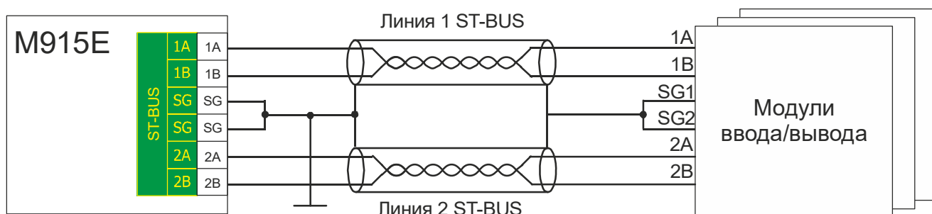
Рисунок 6 - Варианты подключение внешних цепей к юниту RS485
