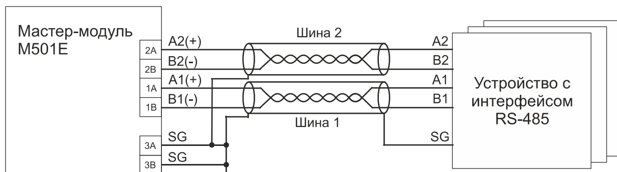
Рисунок 12 - Схема подключения с использованием кабелей с одной витой парой
