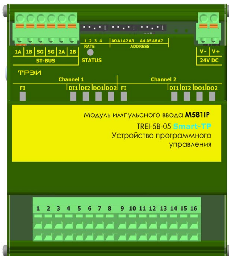
Рисунок 1 - Разъемы и лицевая панель модуля M581IP
