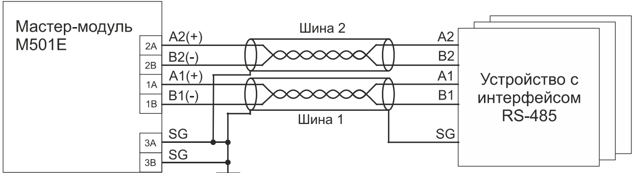
Рисунок 9 - Схема подключения с использованием кабеля с одной витой парой
