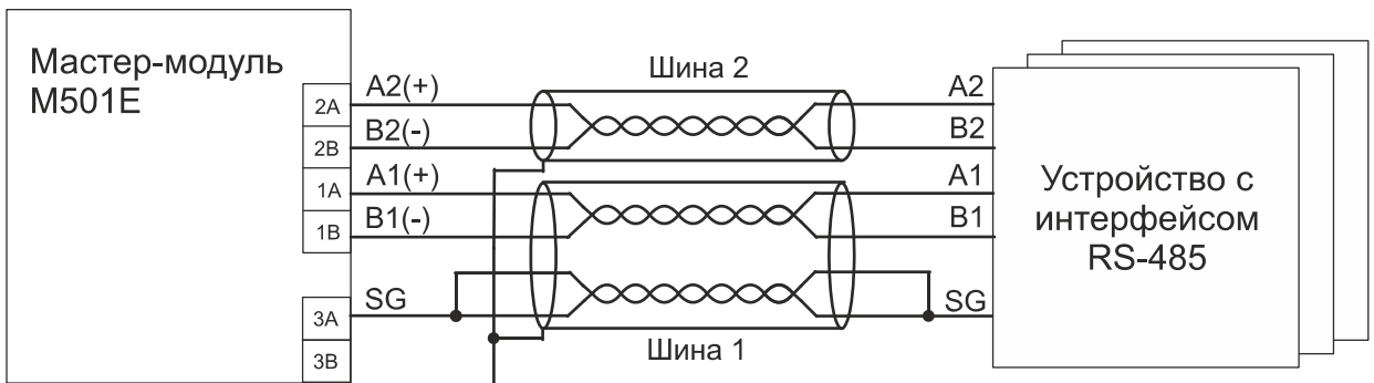
Рисунок 11 - Схема подключения с использованием кабеля с двойной витой парой на одной из шин
