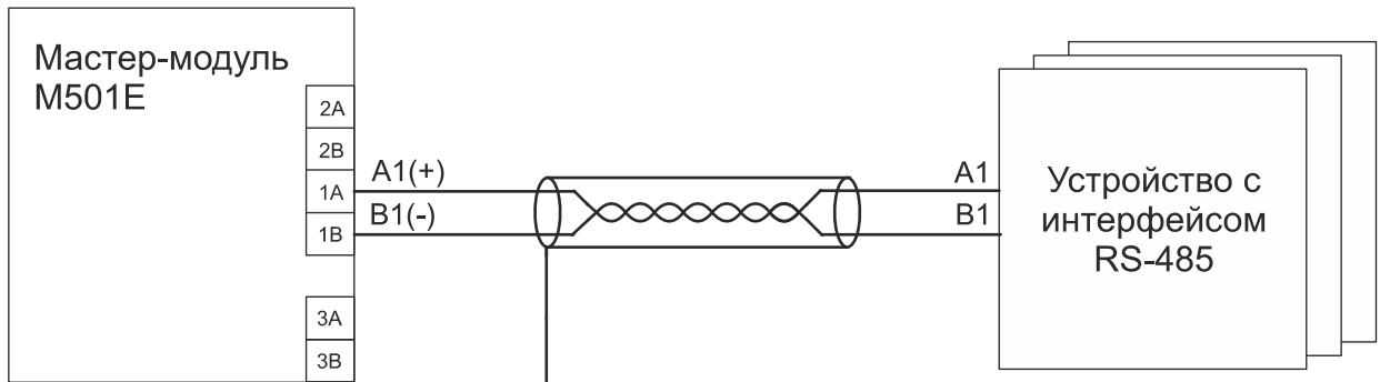
Рисунок 10 - Схема подключения с использованием кабеля с одной витой парой и без клеммы SG
