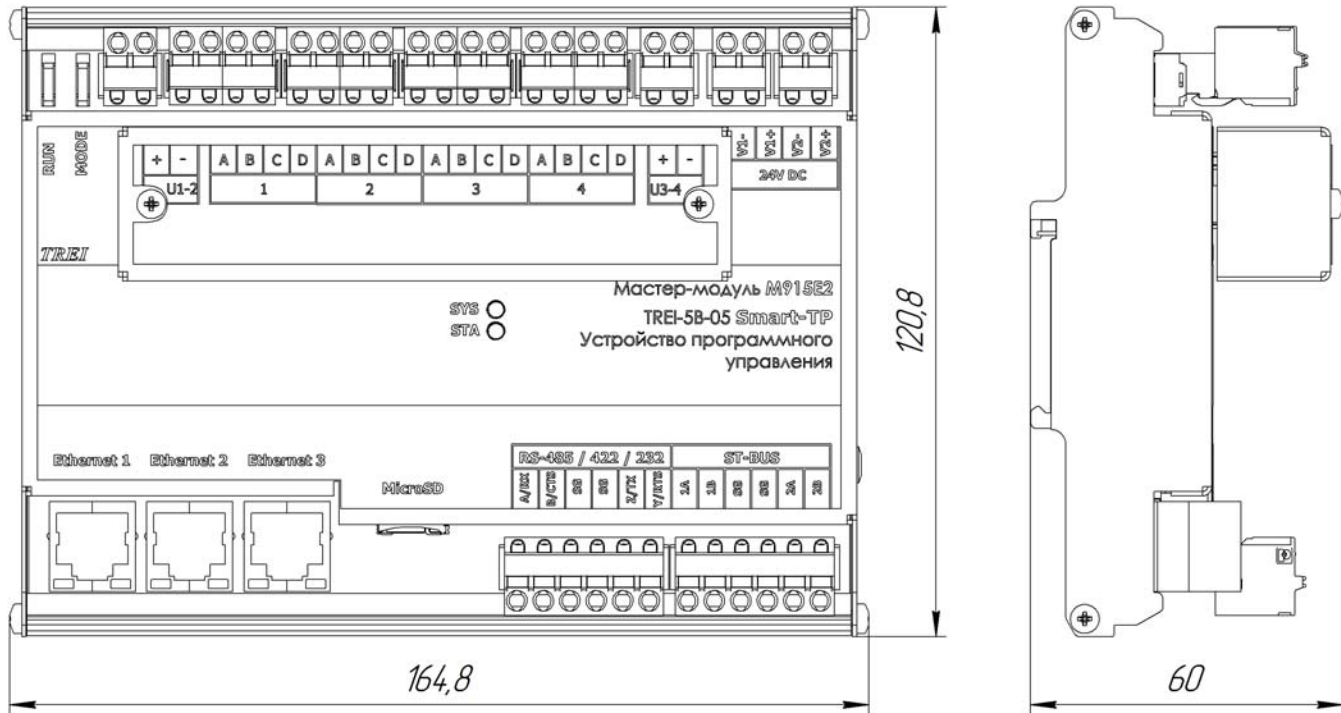
Рисунок 9 - Чертеж общего вида M915E2 с указанием габаритных и присоединительных размеров
