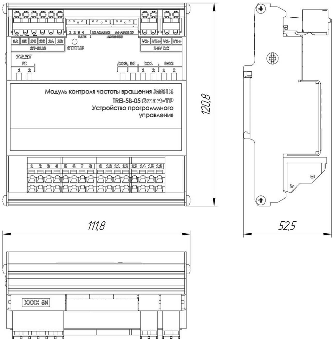
Рисунок 4 - Чертеж общего вида M581IS с указанием габаритных и присоединительных размеров
