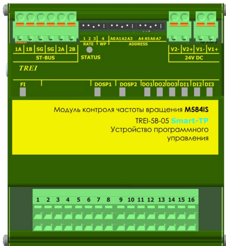
Рисунок 1 - Разъемы и лицевая панель модуля M584IS
