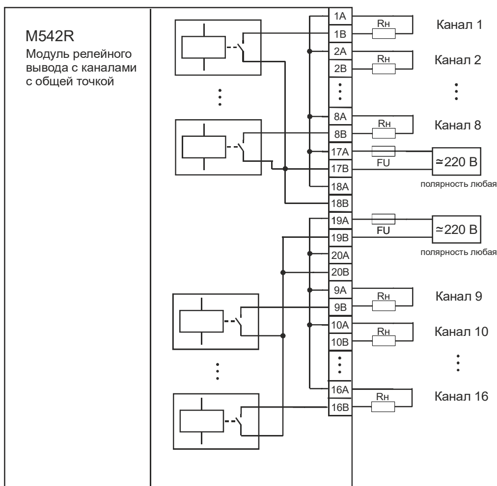
Рисунок 3 - Схема подключения внешних цепей модуля M542R*
