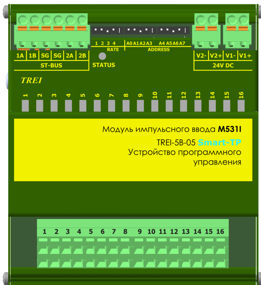
Рисунок 1 - Разъемы и лицевая панель модуля M5311
