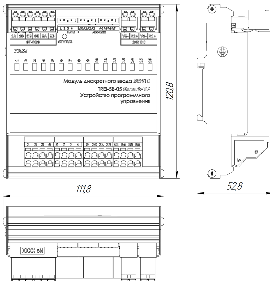
Рисунок 3 - Чертеж общего вида M541D с указанием габаритных и присоединительных размеров
