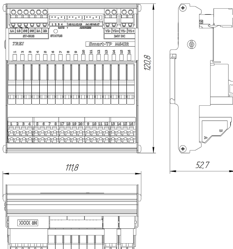
Рисунок 4 - Чертеж общего вида M542R с указанием габаритных и присоединительных размеров
