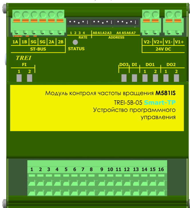
Рисунок 1 - Разъемы и лицевая панель модуля M581IS
