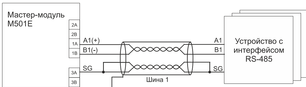
Рисунок 6 - Схема подключения с использованием кабеля с двойной витой парой
