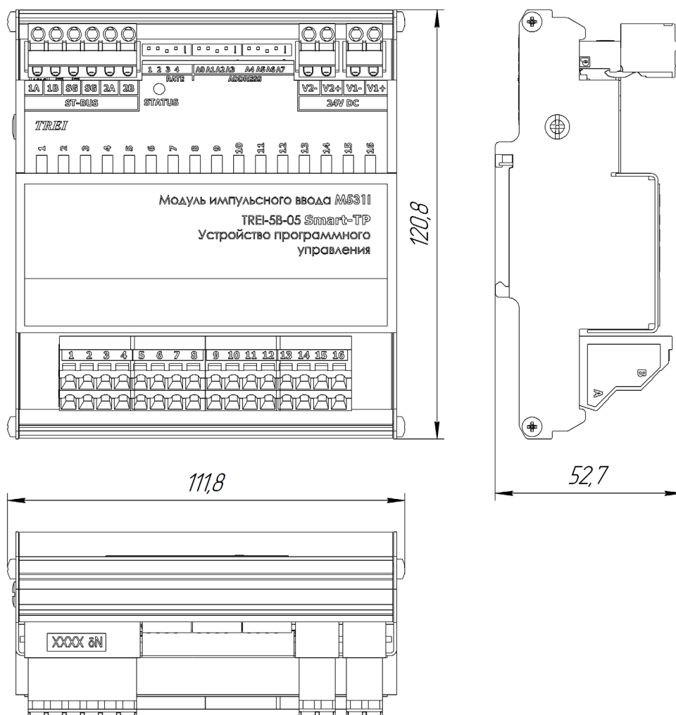
Рисунок 3 - Чертеж общего вида M5311 с указанием габаритных и присоединительных размеров
