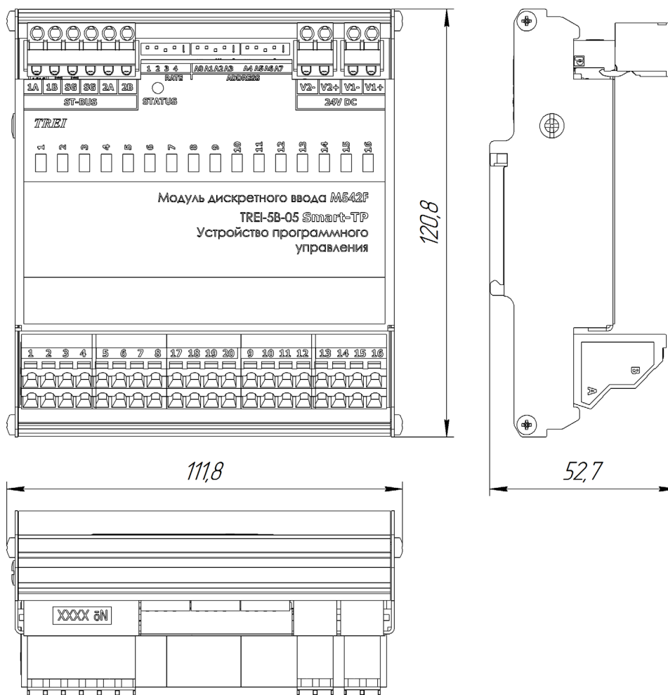
Рисунок 3 - Чертеж общего вида M542F с указанием габаритных и присоединительных размеров
