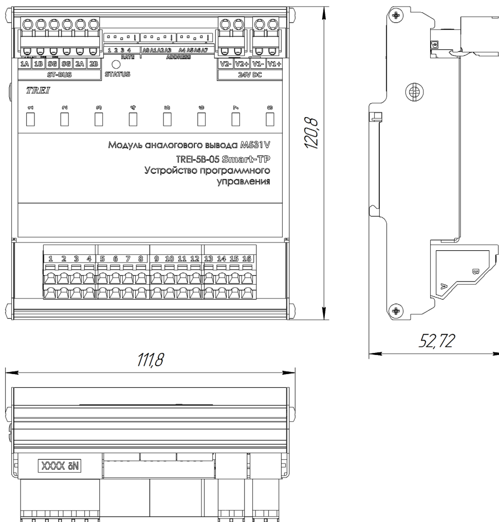
Рисунок 2 - Чертеж общего вида M531V с указанием габаритных и присоединительных размеров
