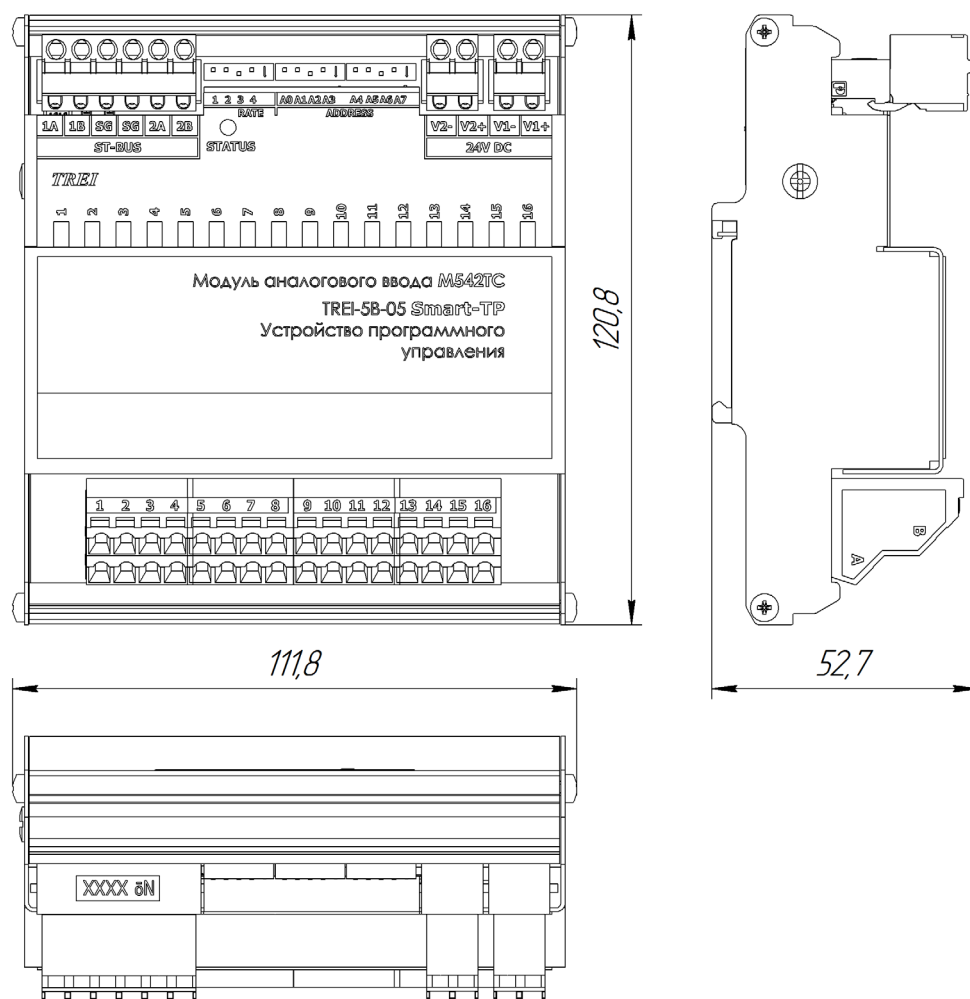
Рисунок 2 - Чертеж общего вида M542TC с указанием габаритных и присоединительных размеров
