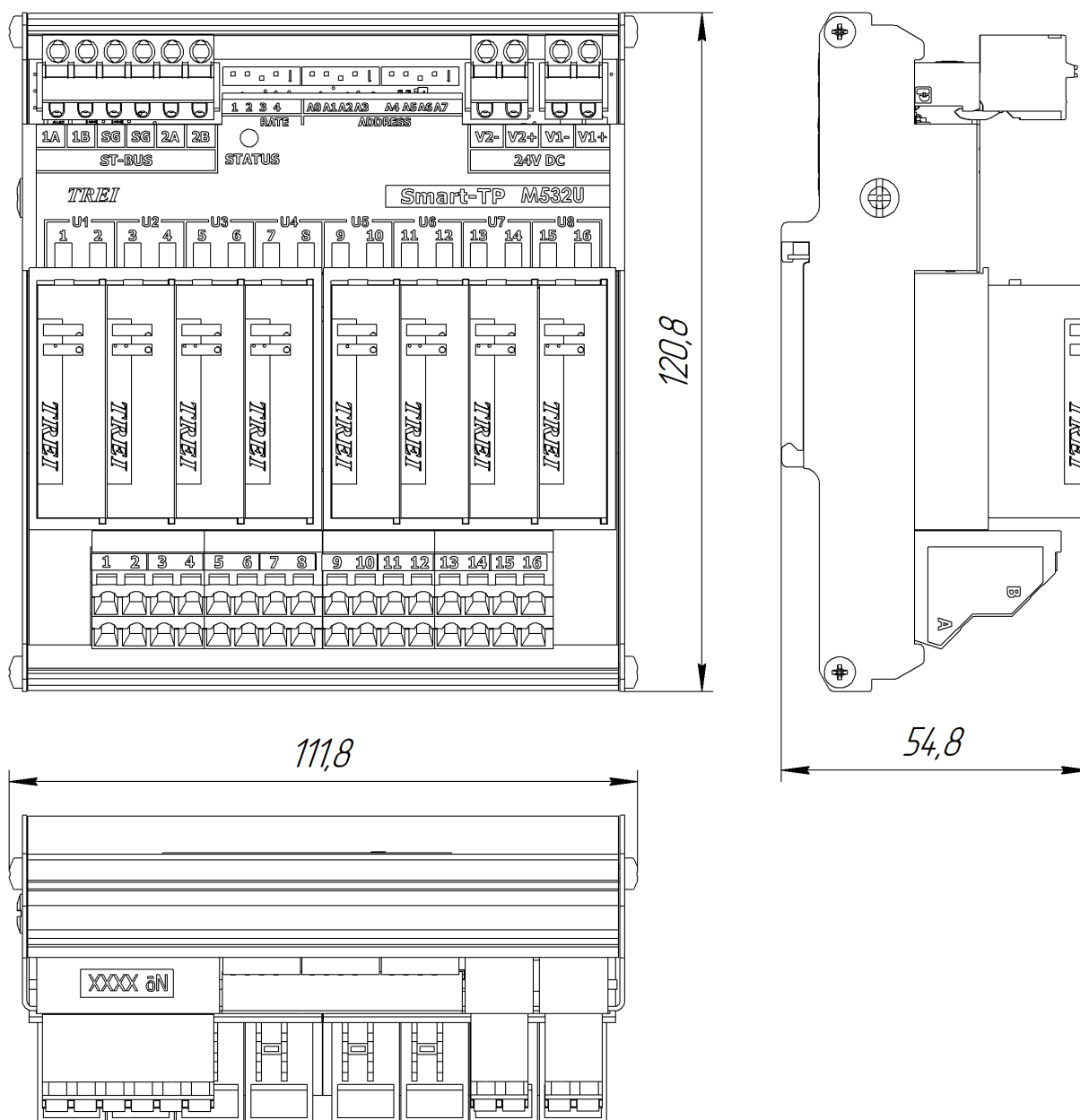
Рисунок 2 - Чертеж общего вида M532U с указанием габаритных и присоединительных размеров
