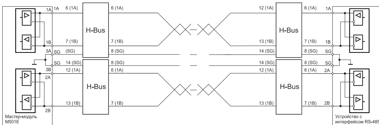
Рисунок 11 - Схема подключения с использованием блока согласования H-BUS
