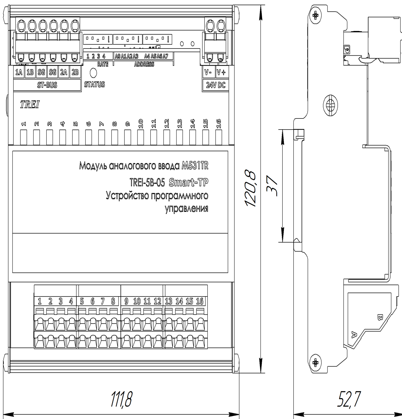
Рисунок 2 - Чертеж общего вида M531TR с указанием габаритных и присоединительных размеров
