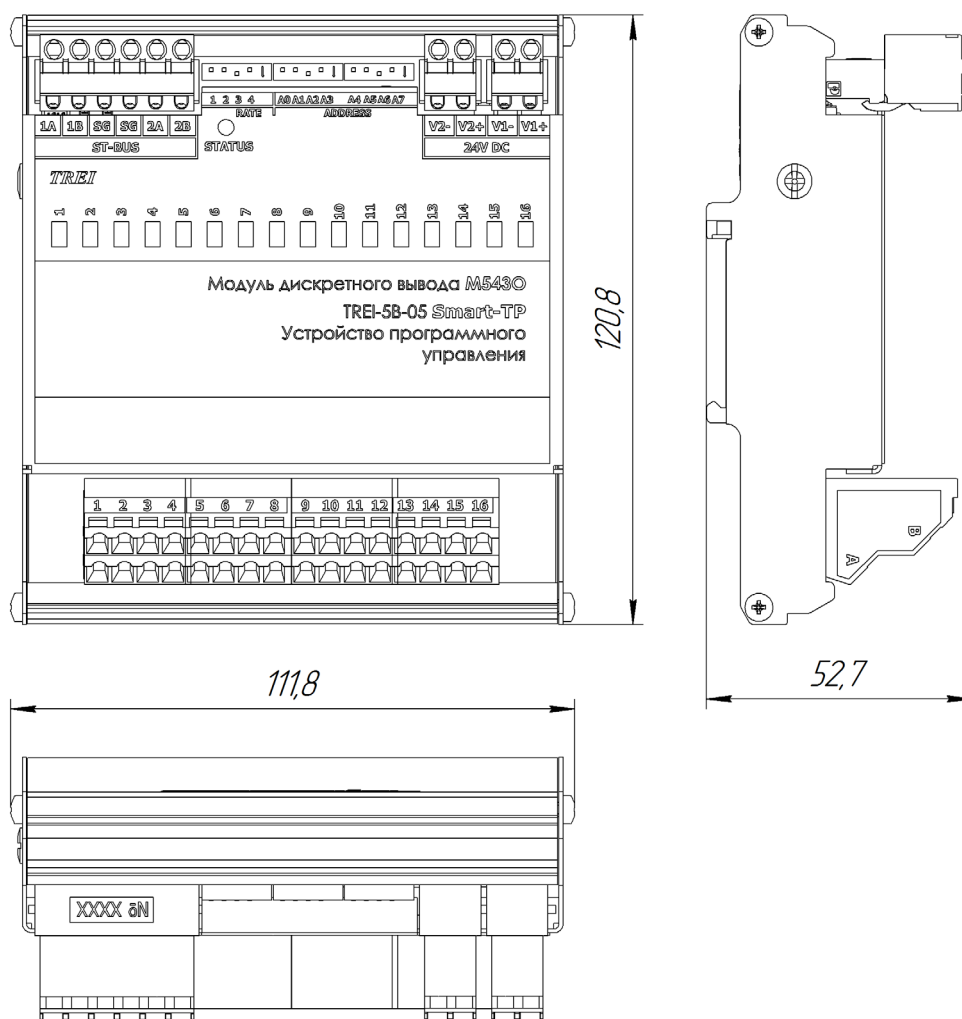
Рисунок 2 - Чертеж общего вида M543O с указанием габаритных и присоединительных размеров
