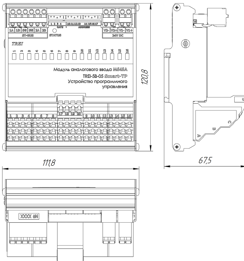
Рисунок 2 - Чертеж общего вида M545A с указанием габаритных и присоединительных размеров
