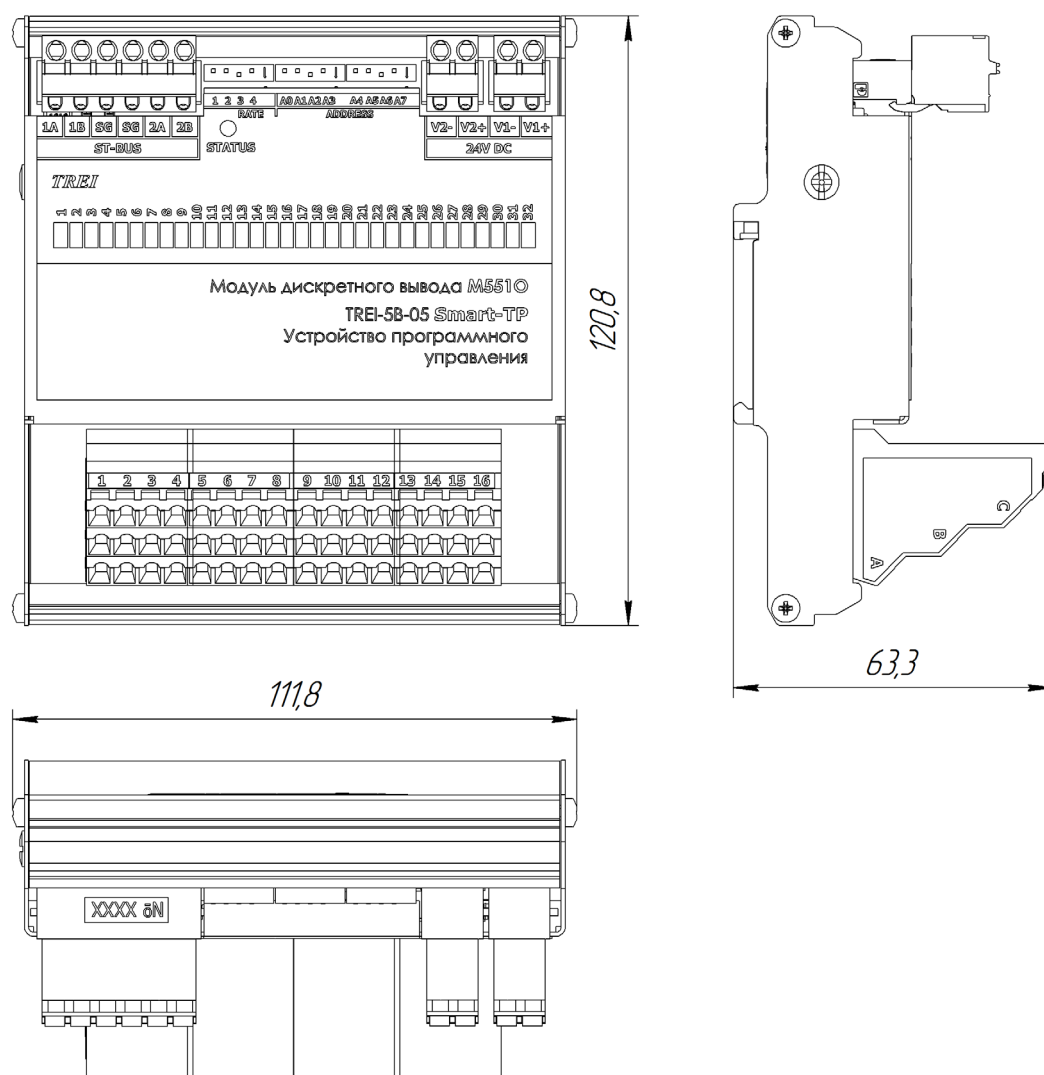
Рисунок 2 - Чертеж общего вида M551O с указанием габаритных и присоединительных размеров
