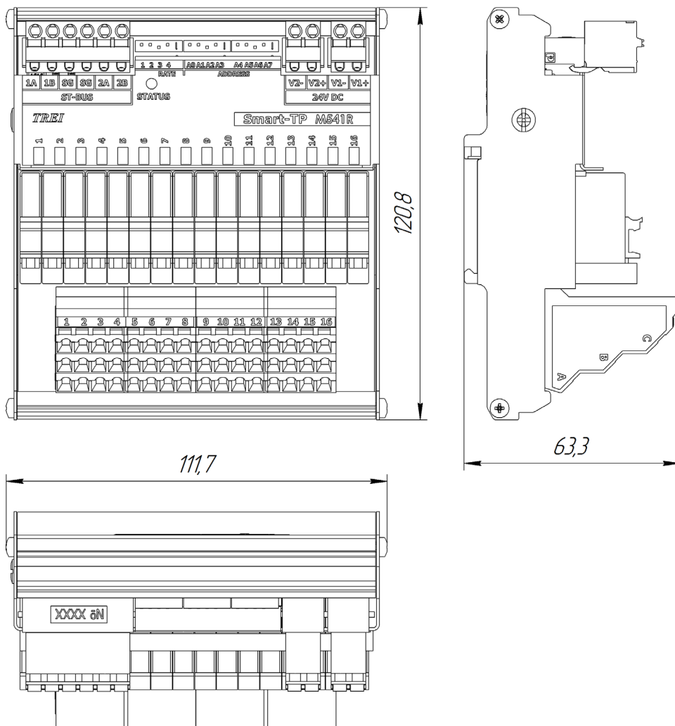
Рисунок 3 - Чертеж общего вида M541R с указанием габаритных и присоединительных размеров
