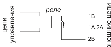
Рисунок 4 - Структура канала юнита релейного вывода с переключающими контактами
