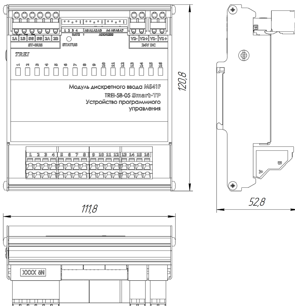
Рисунок 3 - Чертеж общего вида M541F с указанием габаритных и присоединительных размеров
