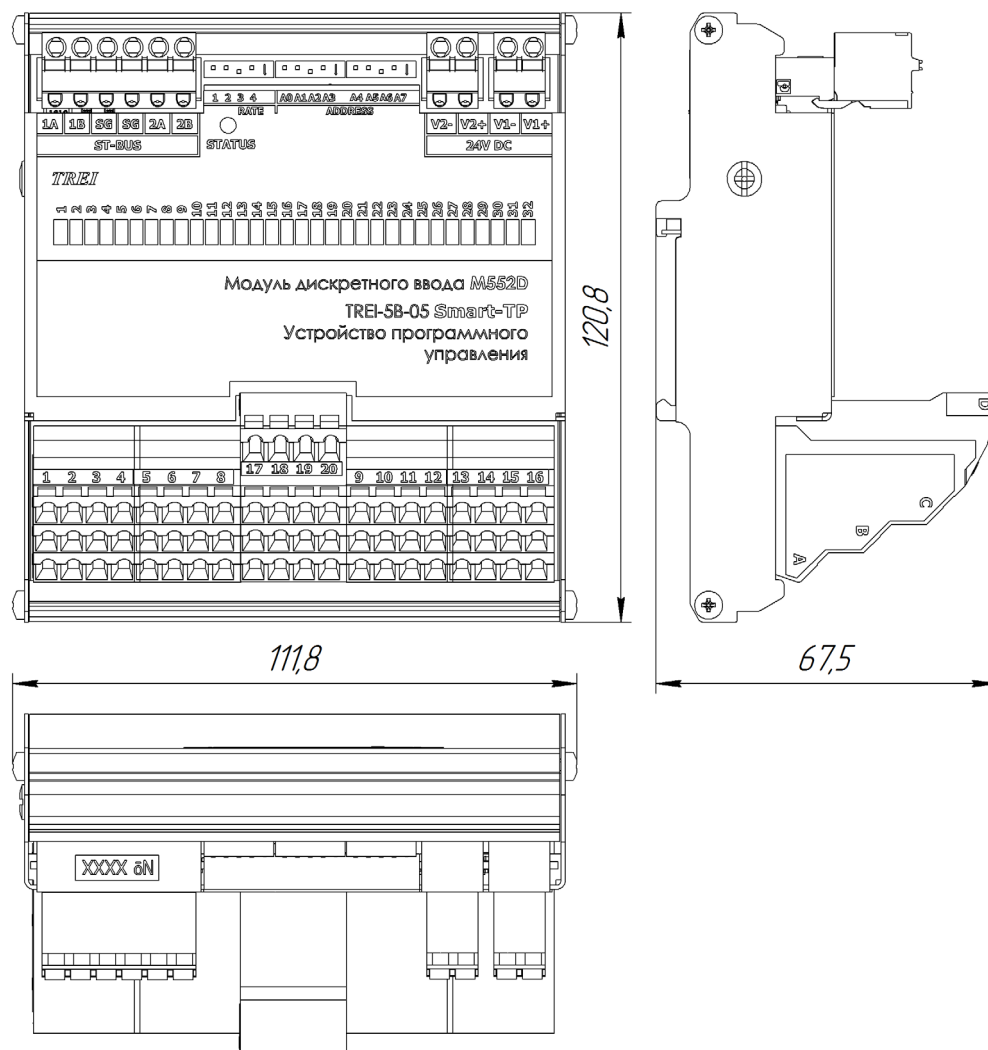
Рисунок 2 - Чертеж общего вида M552D с указанием габаритных и присоединительных размеров
