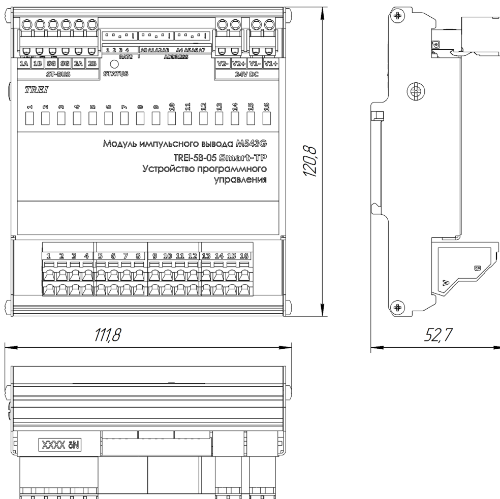
Рисунок 2 - Чертеж общего вида M543G с указанием габаритных и присоединительных размеров
