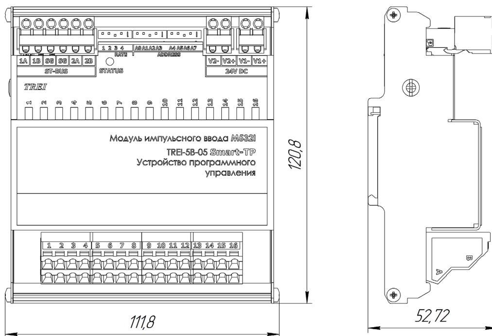
Рисунок 4 - Чертеж общего вида M532I с указанием габаритных и присоединительных размеров
