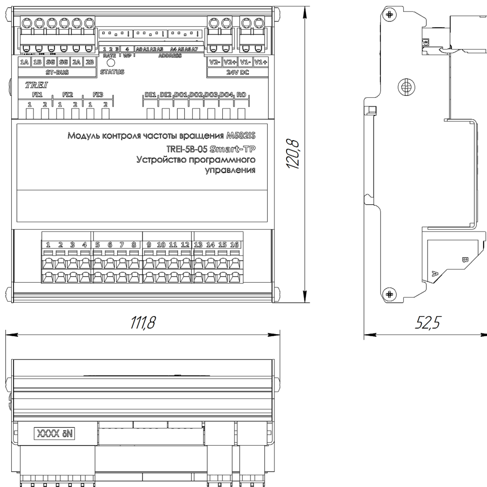
Рисунок 3 - Чертеж общего вида M582IS с указанием габаритных и присоединительных размеров
