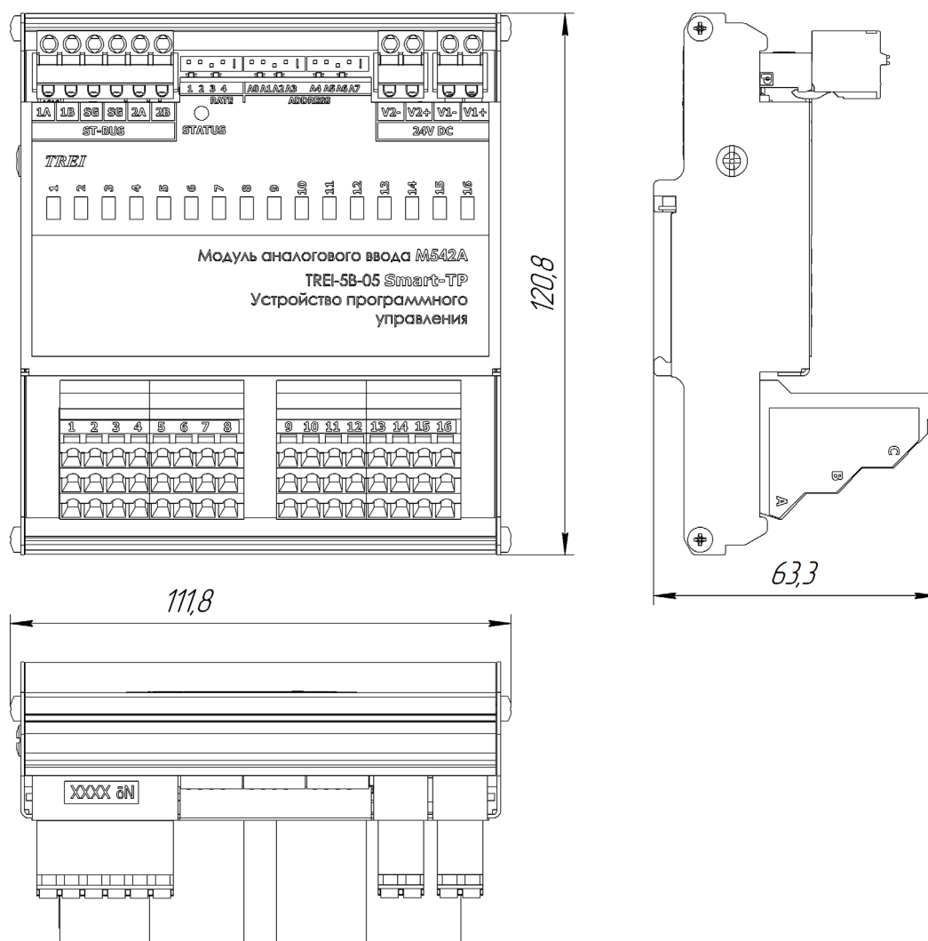
Рисунок 2 - Чертеж общего вида M542A с указанием габаритных и присоединительных размеров
