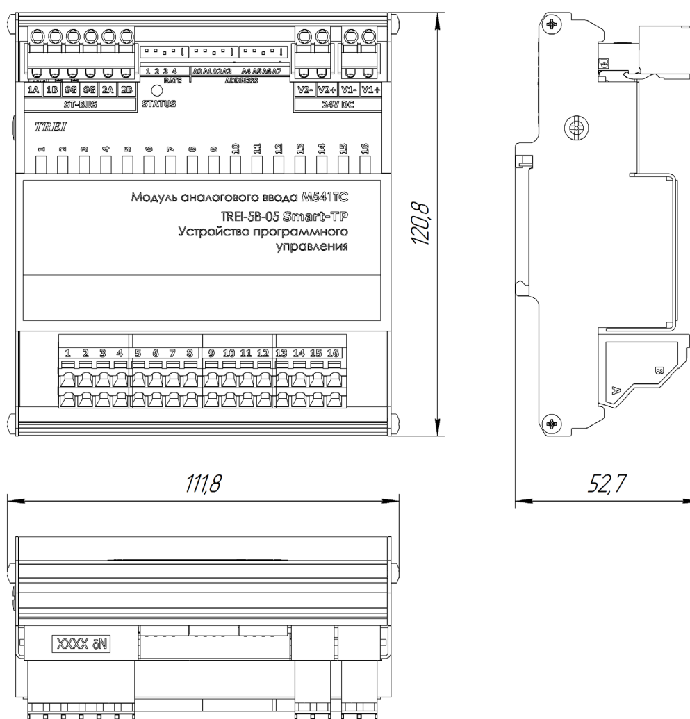
Рисунок 2 - Чертеж общего вида M541TC с указанием габаритных и присоединительных размеров
