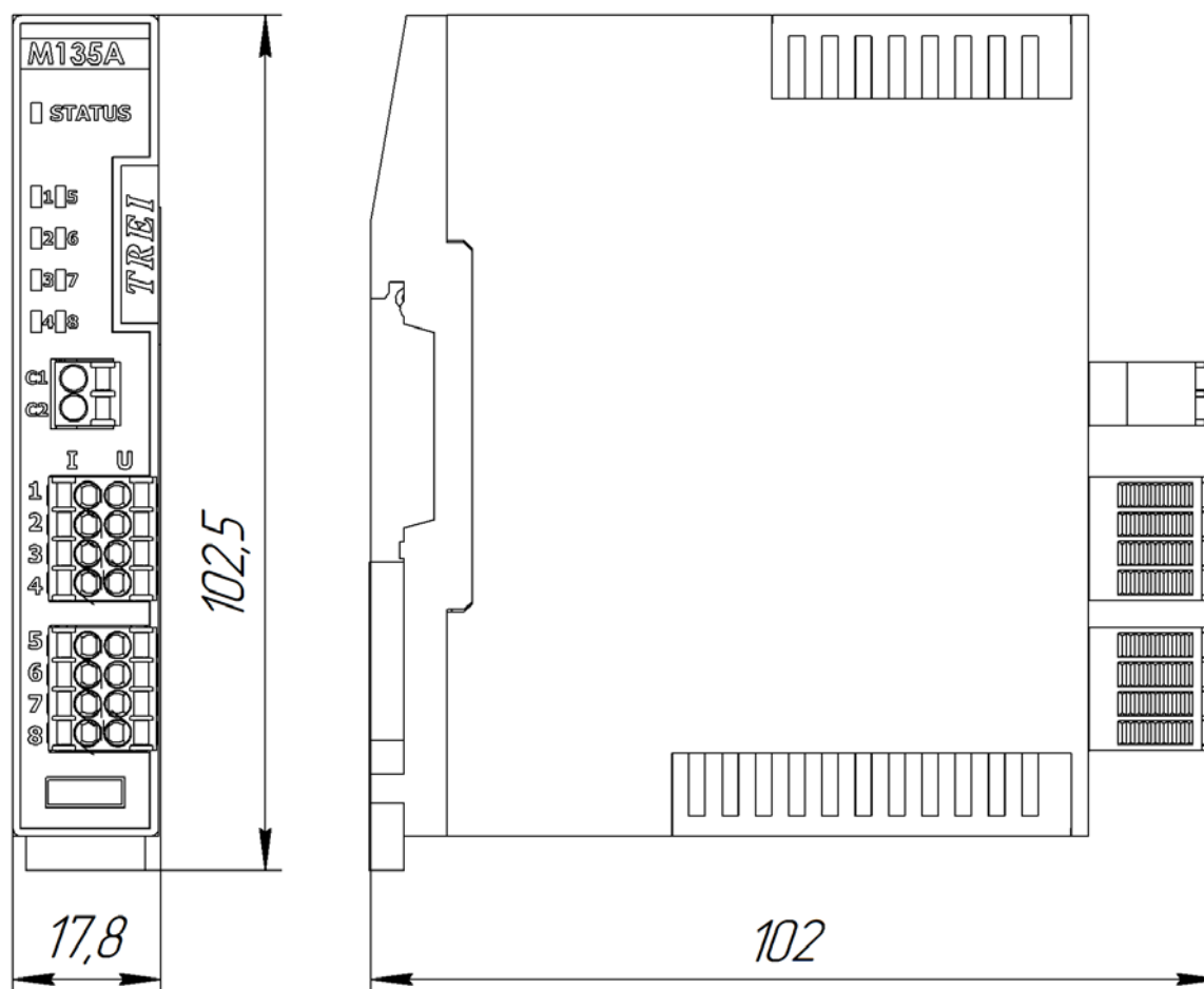
Рисунок 3 - Чертеж общего вида M135A с указанием габаритных и присоединительных размеров
