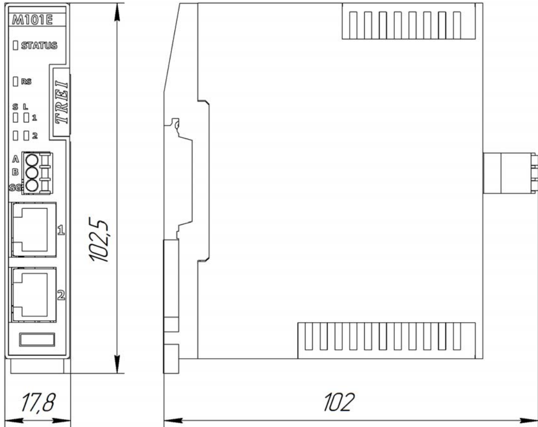
Рисунок 4 - Чертеж общего вида M101E с указанием габаритных и присоединительных размеров
