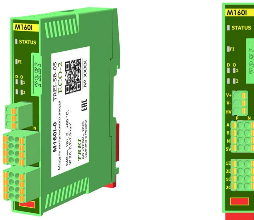
Рисунок 1 - Разъемы и лицевая панель модуля M160I
