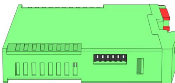
Рисунок 2 - расположение переключателя "ADDRESS"
