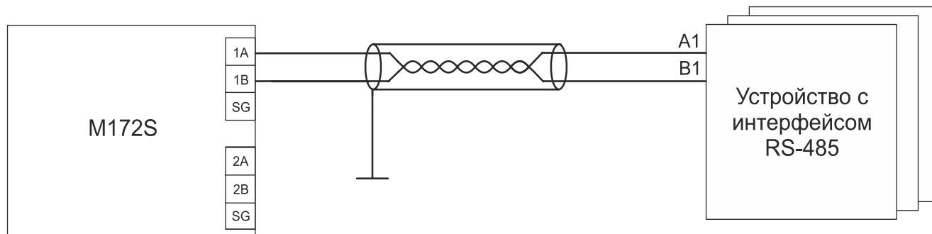
Рисунок 4 - Схема подключения с использованием кабеля "витая пара" и без клеммы SG
