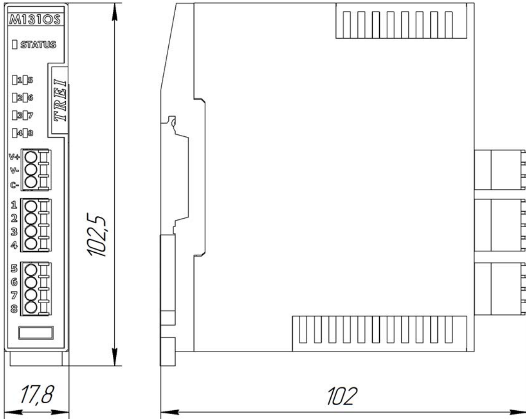
Рисунок 3 - Чертеж общего вида M131O, M131OS с указанием габаритных и присоединительных размеров
