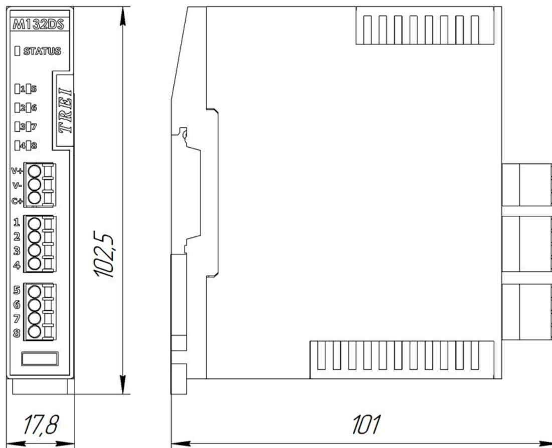
Рисунок 3 - Чертеж общего вида M132D, M132DS с указанием габаритных и присоединительных размеров
