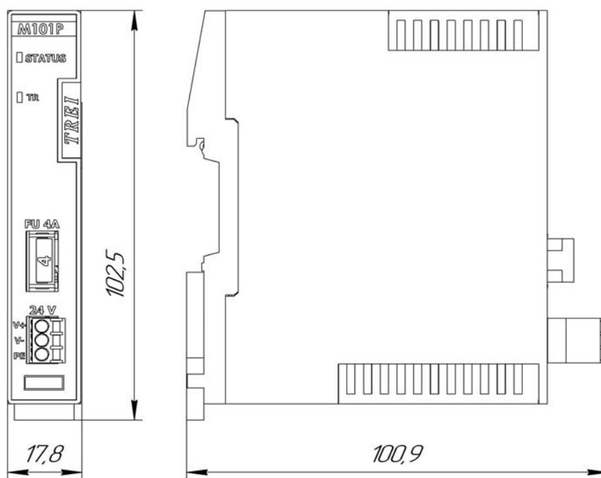
Рисунок 3 - Чертеж общего вида M101P с указанием габаритных и присоединительных размеров
