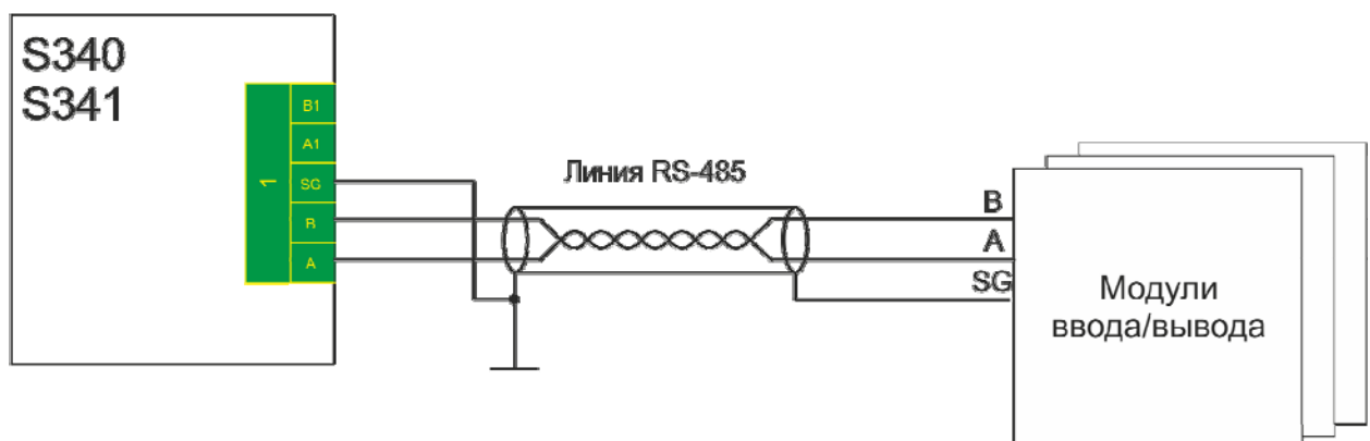
канал RS-485 (полудуплекс)
