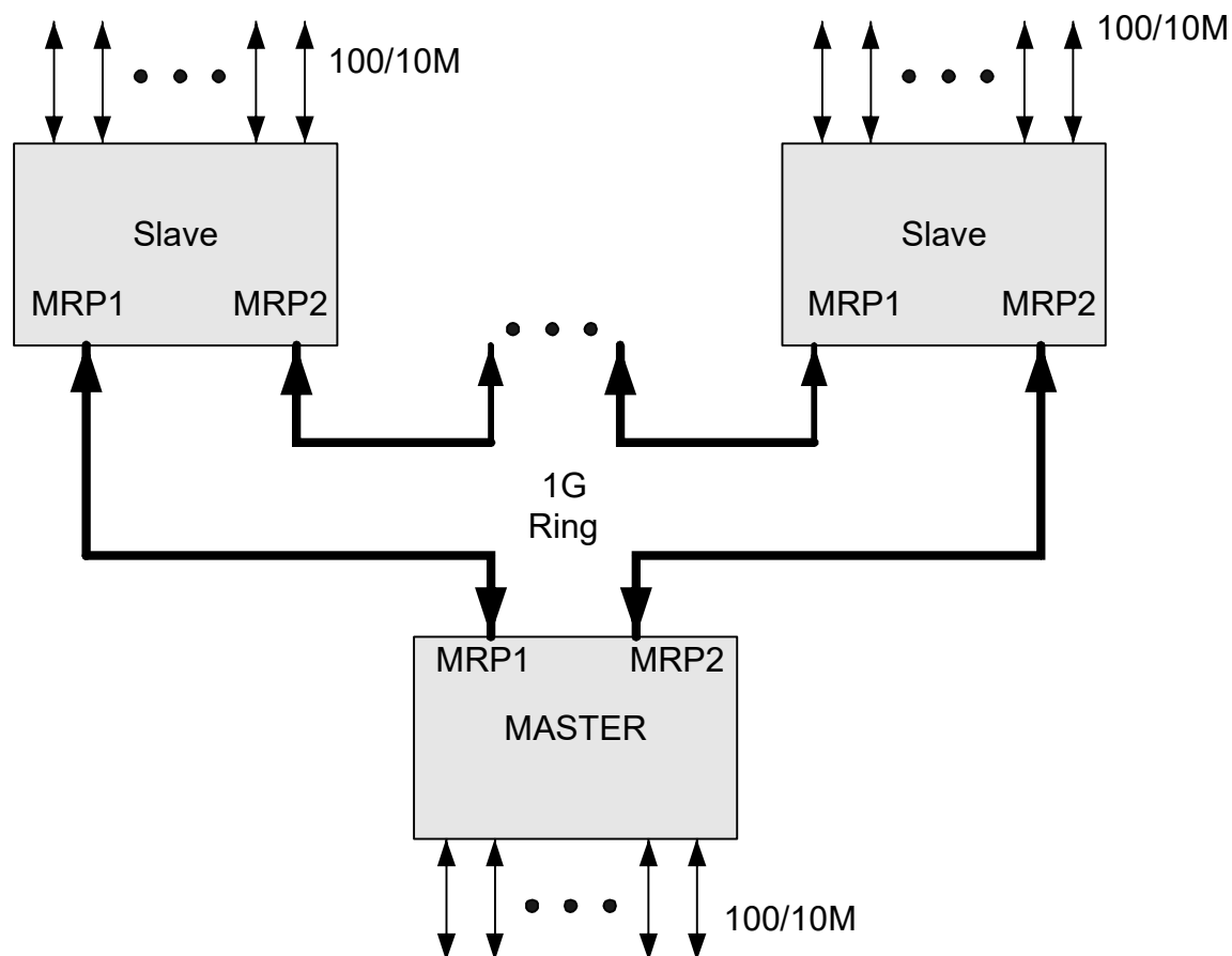
Рисунок 3 - Топология MRP
