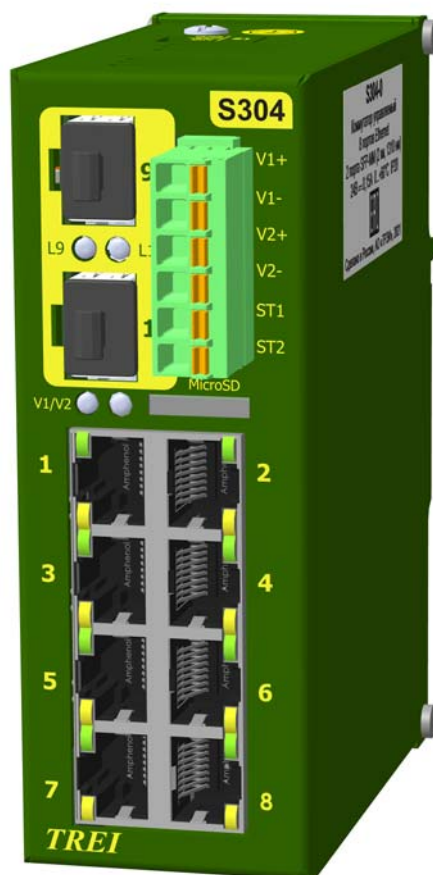
Рисунок 1 - Общий вид коммутатора S304
