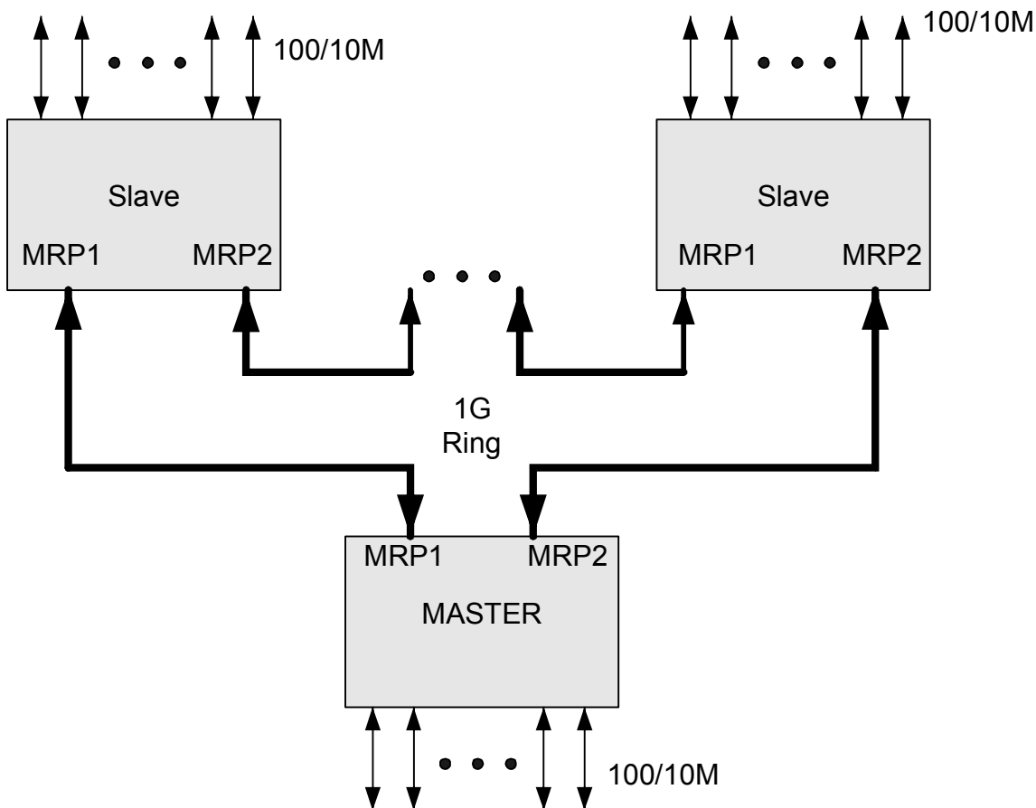
Рисунок 3 - Топология MRP
