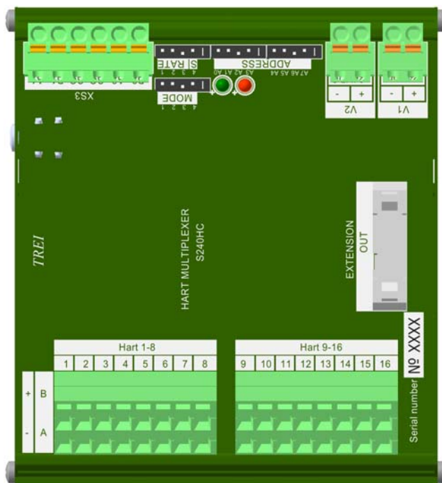
Рисунок 4 - Лицевая панель модуля-мультиплексора HART S240HC
