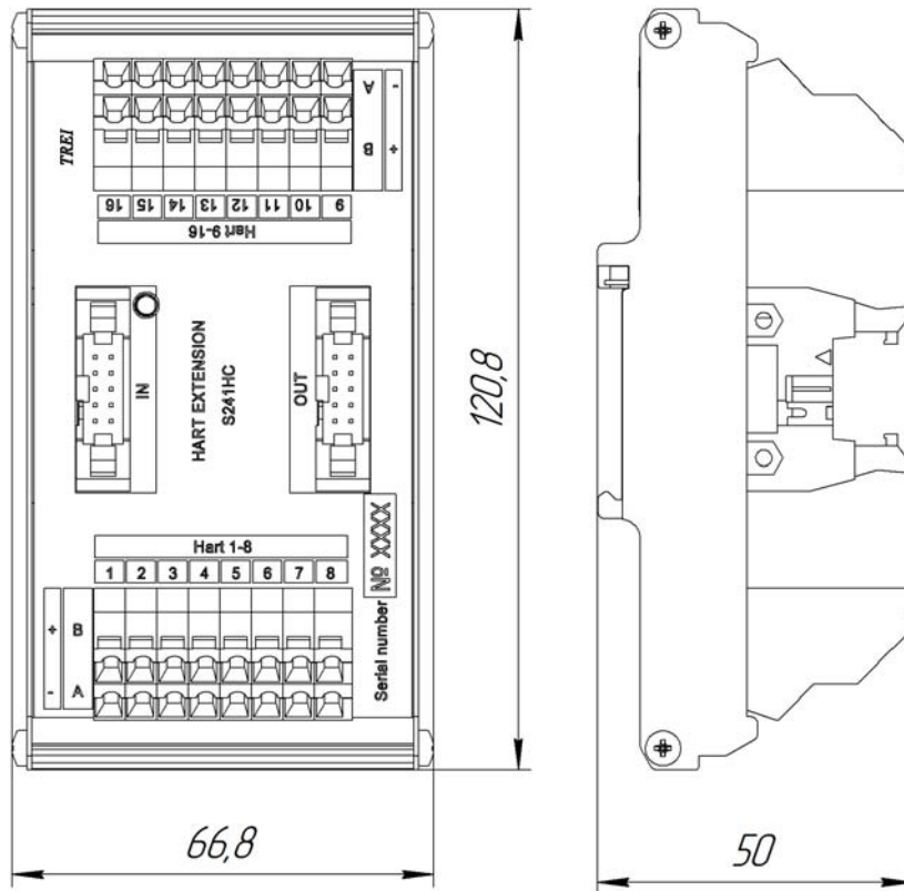
Рисунок 20 - Чертеж общего вида S241HC с указанием габаритных и присоединительных размеров
