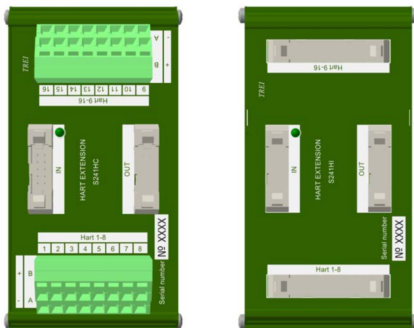
Рисунок 6 - Лицевые панели модулей расширения HART S241HC, S241HI
