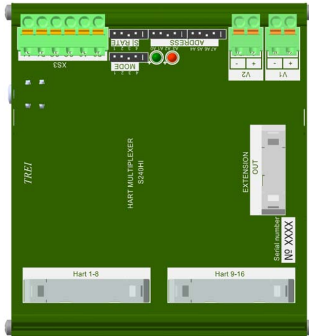
Рисунок 5 - Лицевая панель модуля-мультиплексора HART S240HI
