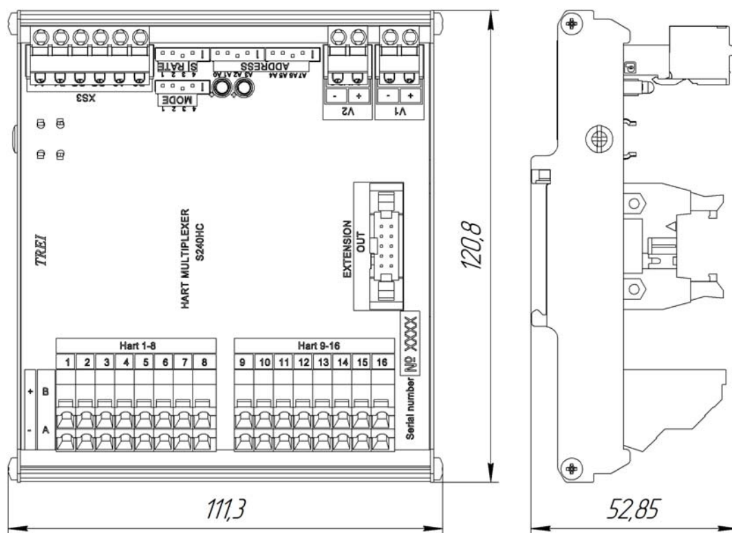
Рисунок 18 - Чертеж общего вида S240HC с указанием габаритных и присоединительных размеров
