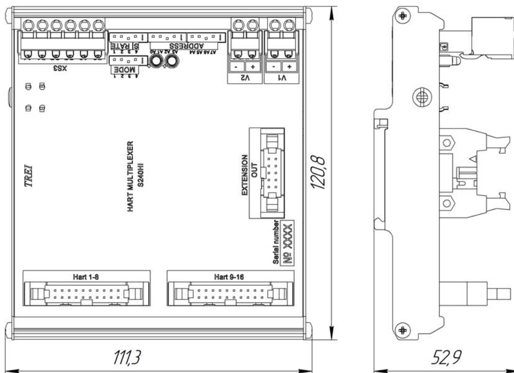
Рисунок 19 - Чертеж общего вида S240HI с указанием габаритных и присоединительных размеров
