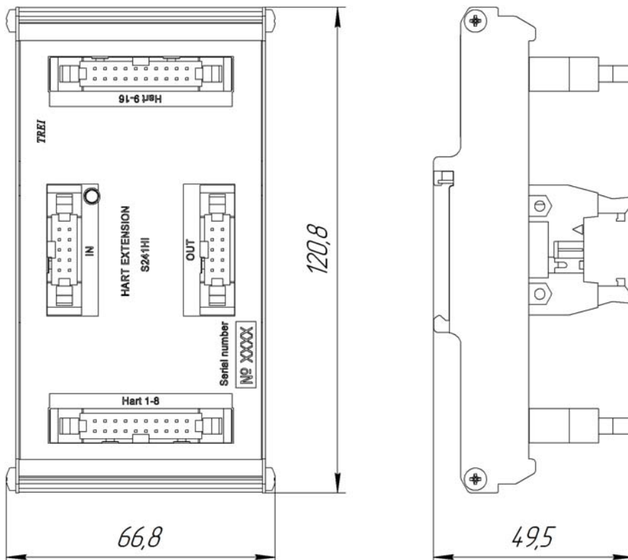
Рисунок 21 - Чертеж общего вида S241HI с указанием габаритных и присоединительных размеров
