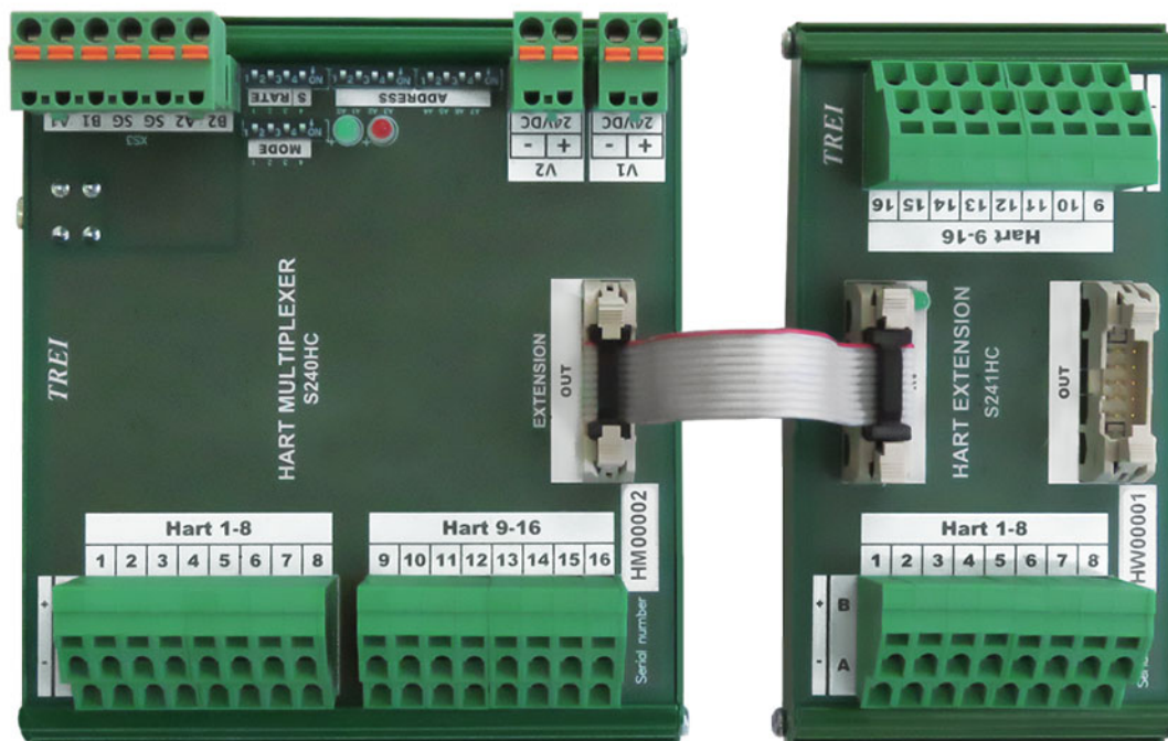
Рисунок 2 - Подключение модулей S240HC, S241HC между собой
