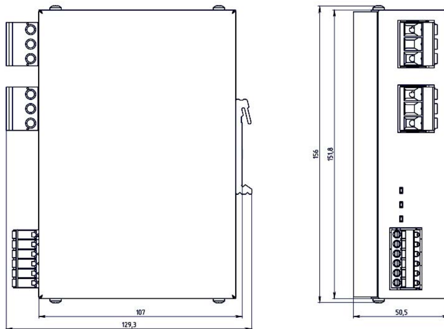
Рисунок 3 - Чертеж общего вида PBR-TB
