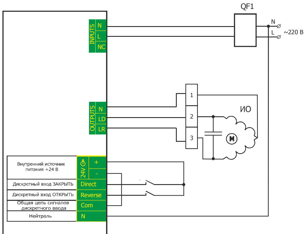
Рисунок 4 - Схема подключения внешних цепей PBR-TB-0X в однофазном исполнении
