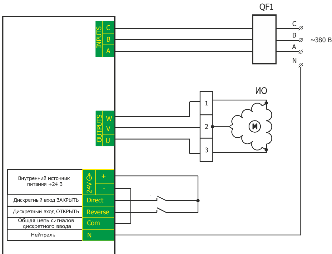
Рисунок 5 - Схема подключения внешних цепей PBR-TB-1X в 3-х фазном исполнении
