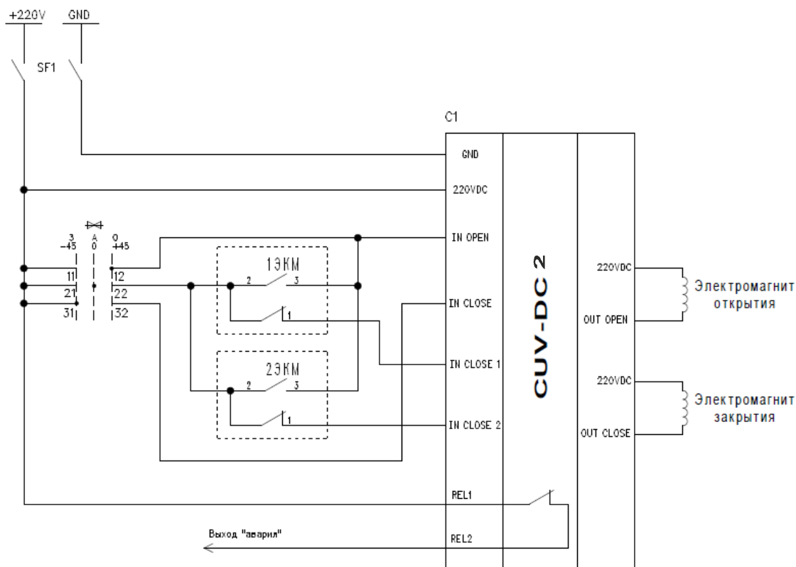
Рисунок 6 – Типовая схема подключения блока CUV-DC 2 с применением ЭКМ
